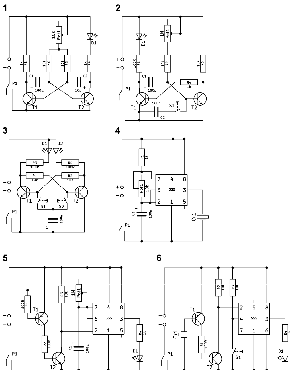
Obr. 40 – Schémata zapojení obvodů z laboratorní práce č. 12
