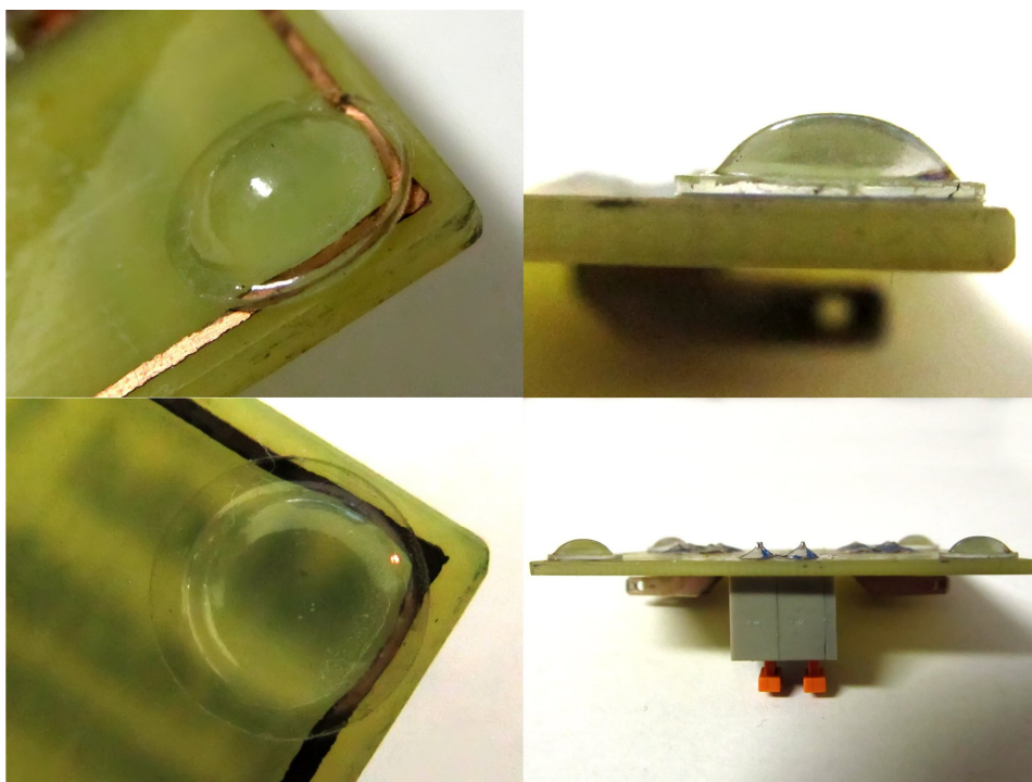
Obr. 3 – Přístrojové nožičky na desce
