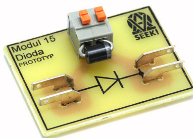
Obr. 23 – Hotový modul (dioda)
