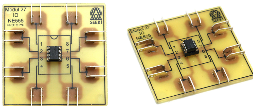
Obr. 28 – Hotový modul (integrovaný obvod NE555)
