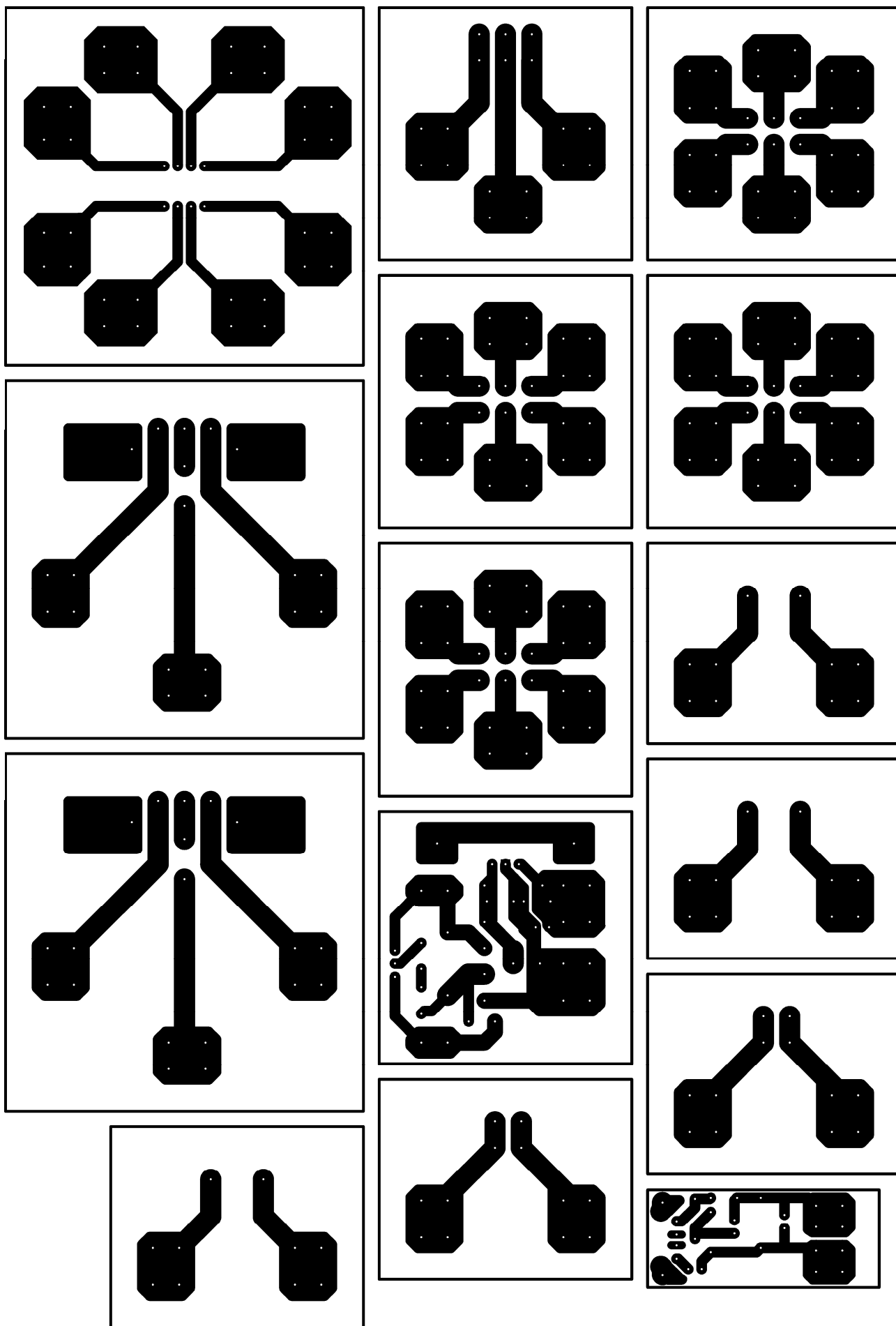
Předloha obrazce plošných spojů druhé desky (šíře 170 mm)
