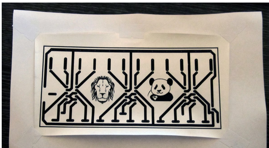
Obr. 6 – Předloha vytištěná na barevném lepicím papíru
