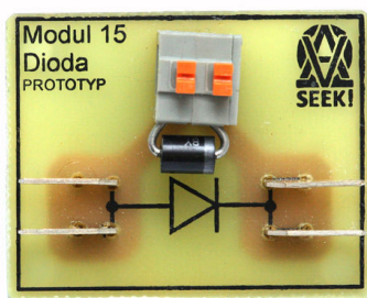
Obr. 23 – Hotový modul (dioda)
