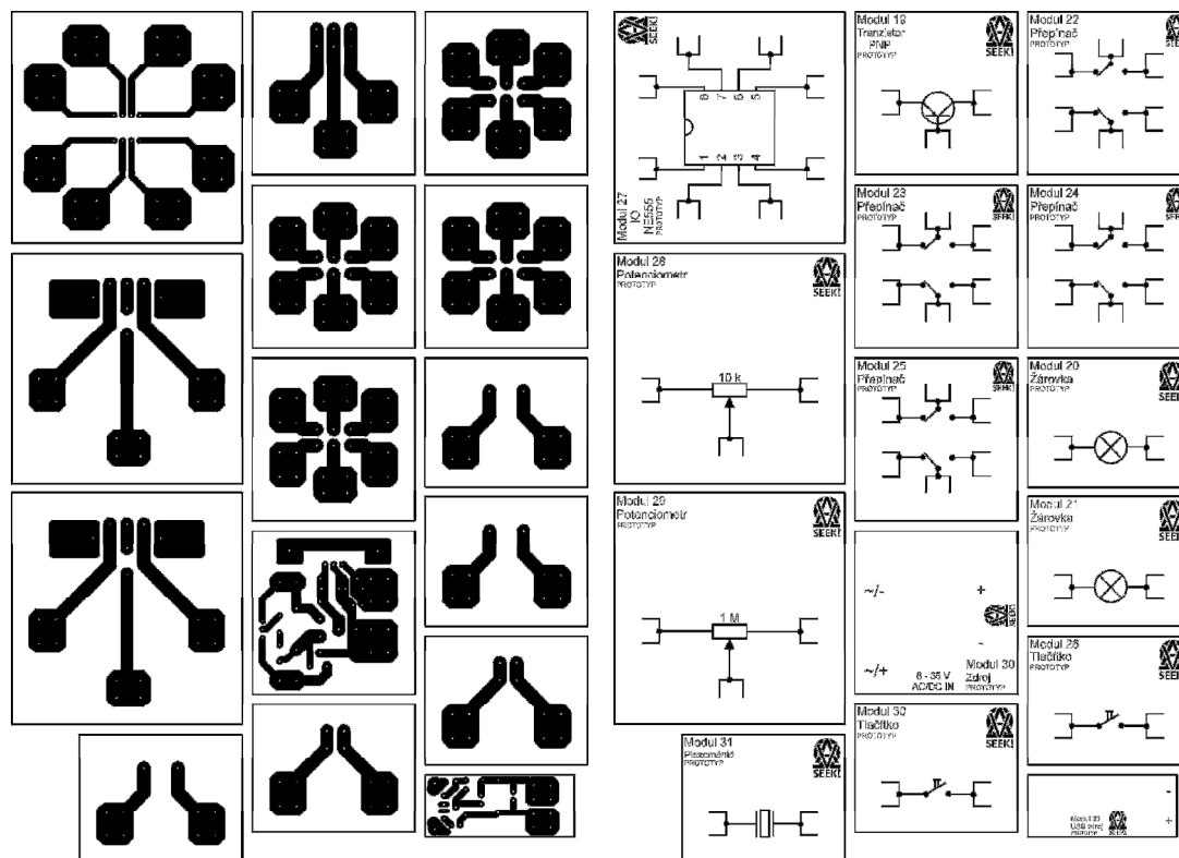
Obr. 17 – Náhledy obrazců spojů a grafiky potisku (deska 2)
