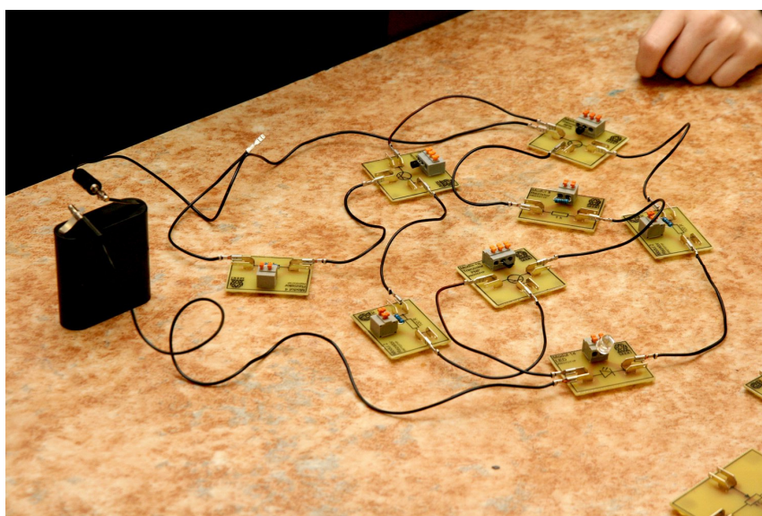
Sestavený obvod třítranzistorového zesilovače
