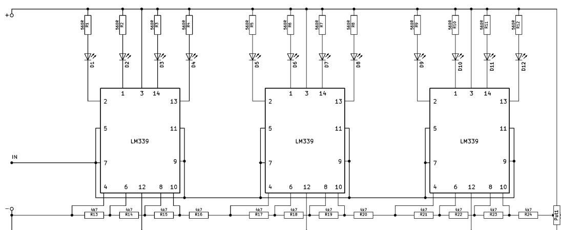
Obr. 4 – Schéma zapojení LED bargrafu
