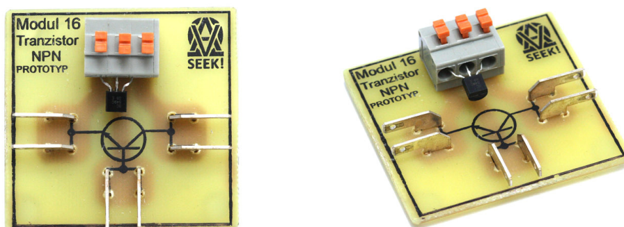
Obr. 24 – Hotový modul (tranzistor)
