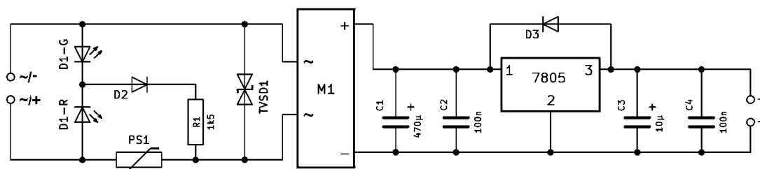
Obr. 32 – Schéma zapojení zdrojového modulu
