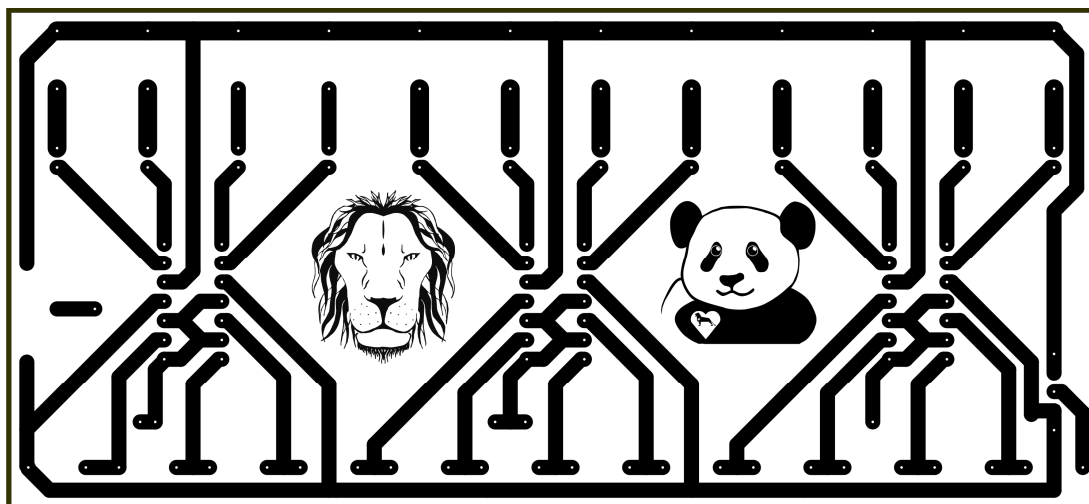
Obr. 5 – Obrazec plošných spojů testovací desky
