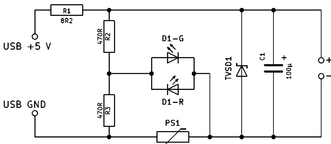
Obr. 34 – Schéma zapojení USB zdrojového modulu
