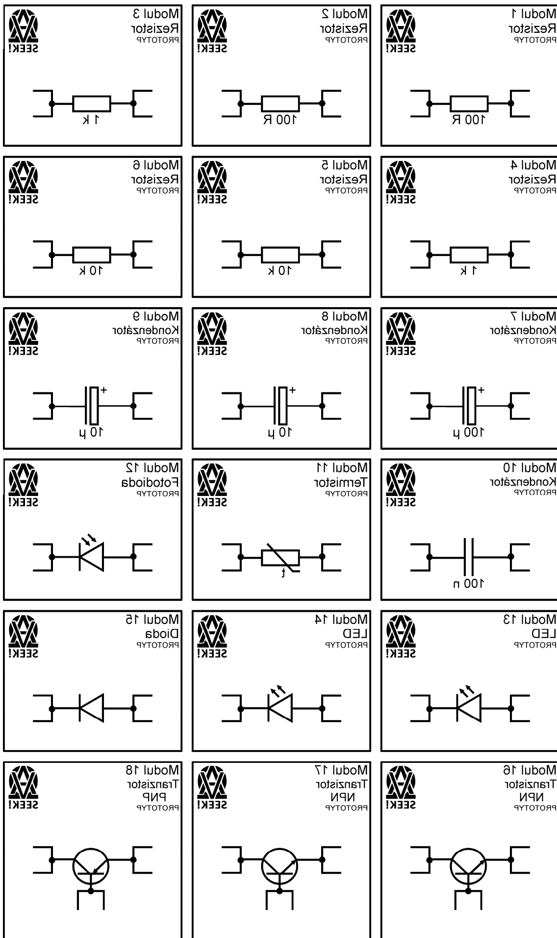
Předloha grafiky první desky (šíře 150 mm)
