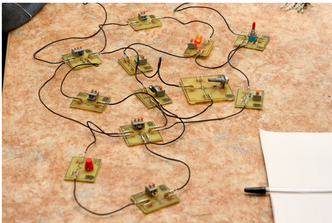
Sestavený monostabilní klopný obvod
