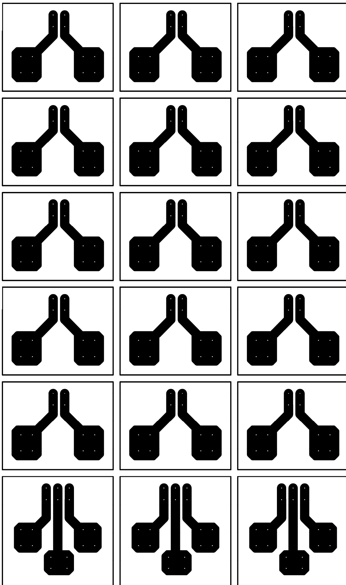
Předloha obrazce plošných spojů první desky (šíře 150 mm)
