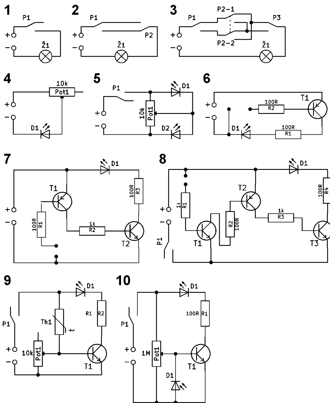
Obr. 38 – Schémata zapojení obvodů z laboratorní práce č. 10
