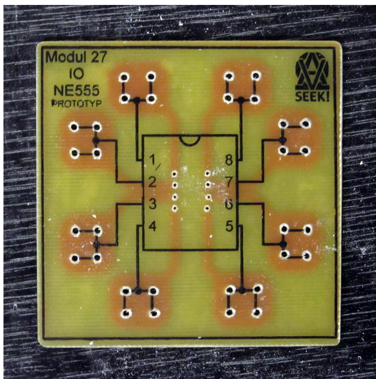
Deska IO NE555 během procesu vrtání
