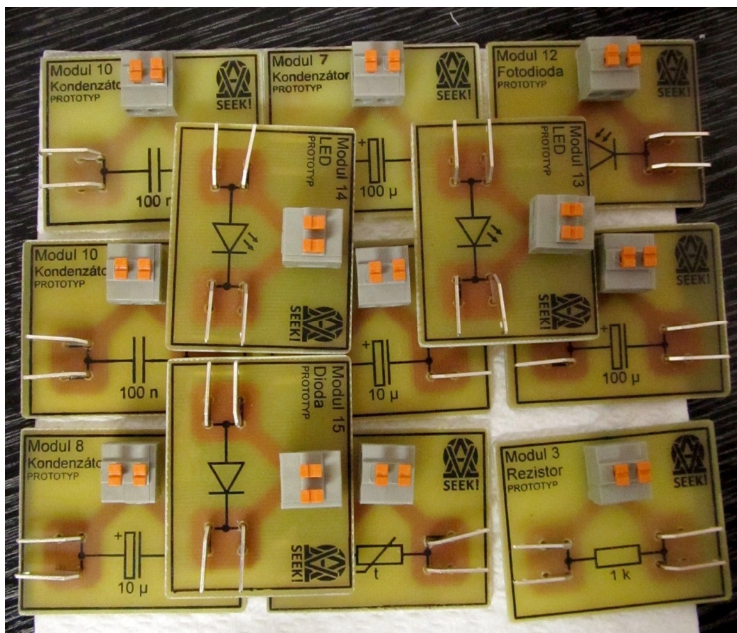
Moduly stavebnice během procesu osazování a pájení
