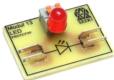
Obr. 22 – Hotový modul (LED)
