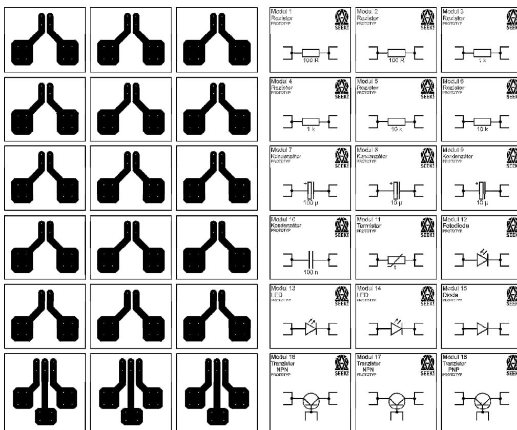
Obr. 16 – Náhledy obrazců spojů a grafiky potisku (deska 1)
