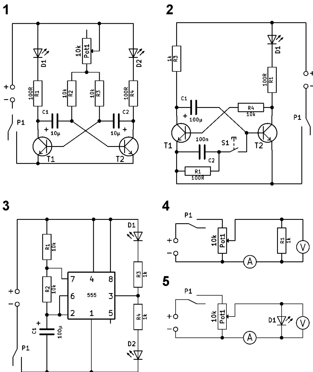
Obr. 39 – Schémata zapojení obvodů z laboratorní práce č. 11
