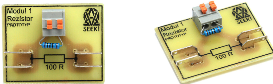
Obr. 18 – Hotový modul (rezistor)
